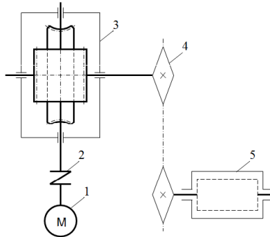
Рисунок 1. Кинематическая схема привода
