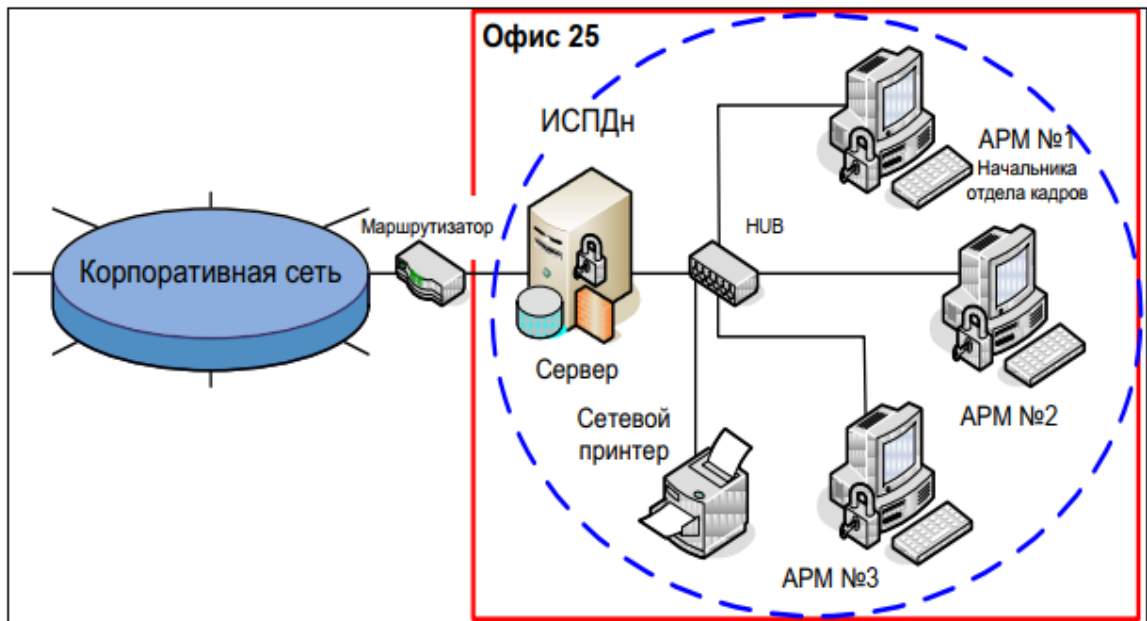
Рис. 7. Схема корпоративной сети
